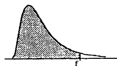
Tavola n. 6.1 Distribuzione cumulativa F di Fisher
